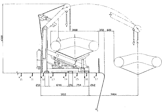
SECTION 7-E 1:50
