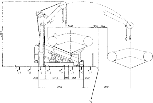
SECTION 7-E 1:50
