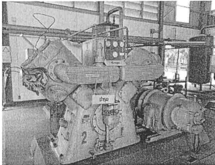
รูปที่ 1 เครื่องอัดลมและอุปกรณ์ประกอบเดิมที่ต้องทำการรื้อถอน
